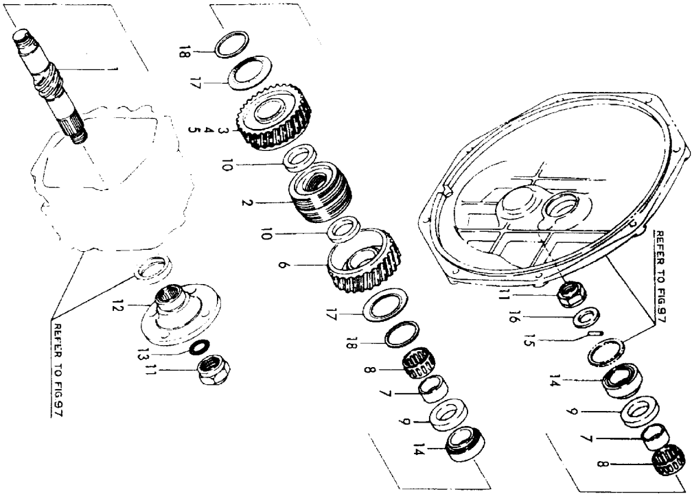
Fig.99 出力シャフト OUTPUT SHAFT
