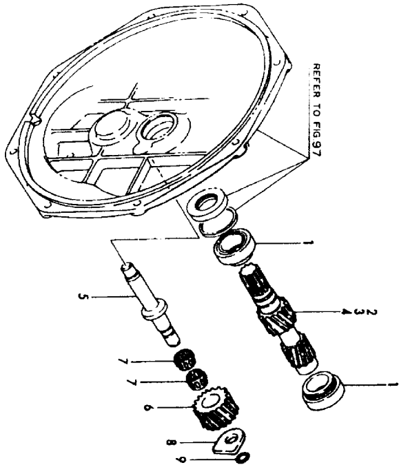
Fig. 98 インプットシャフト & サポートシャフト INPUT SHAFT & SUPPORT SHAFT
