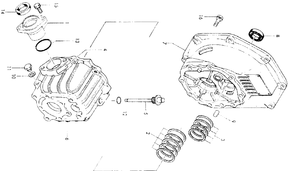
Fig. 102 クラッチケース CLUTCH CASE
