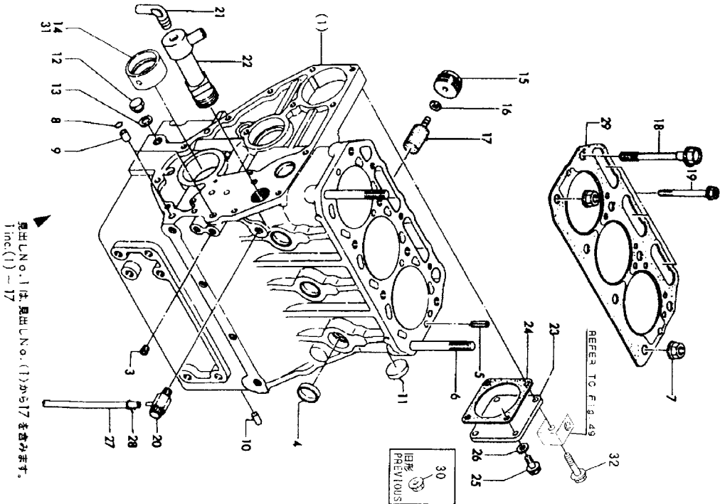
Fig.1 シリンダブロック CYLINDER BLOCK
