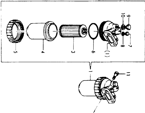
Fig. 46 燃料フィルタ FUEL STRAINER
