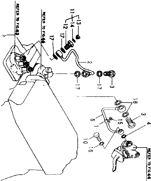
Fig.49 燃料パイプ FUEL PIPE
