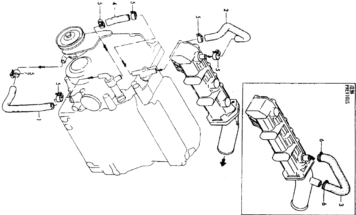
Fig 38 冷却水パイプ(海水) COOLING SEA WATER PIPE
