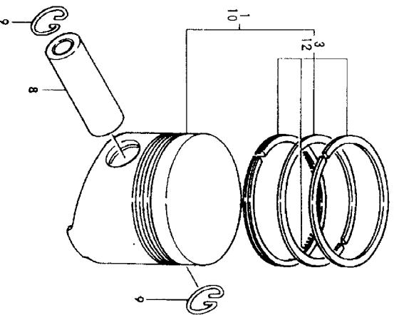
Fig. 25 ピストン PISTON
