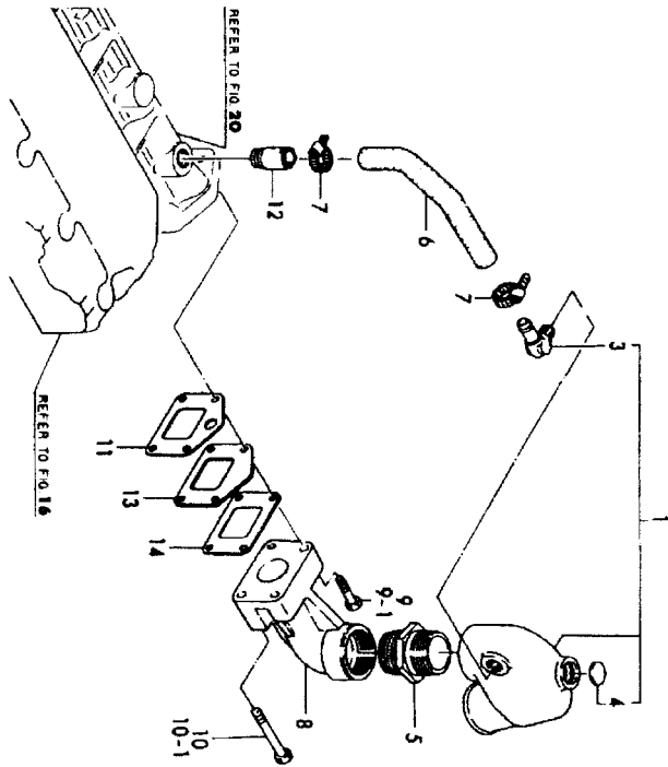
Fig.72 ミキシングエルボ(オプション) MIXING ELBOW(OPTIONAL)
