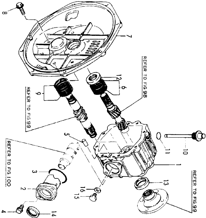
Fig.97 クラッチケース CLUTCH HOUSING
