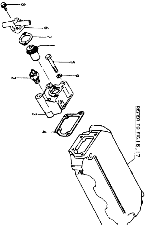
サーモスタット Fig.40 THERMOSTAT
