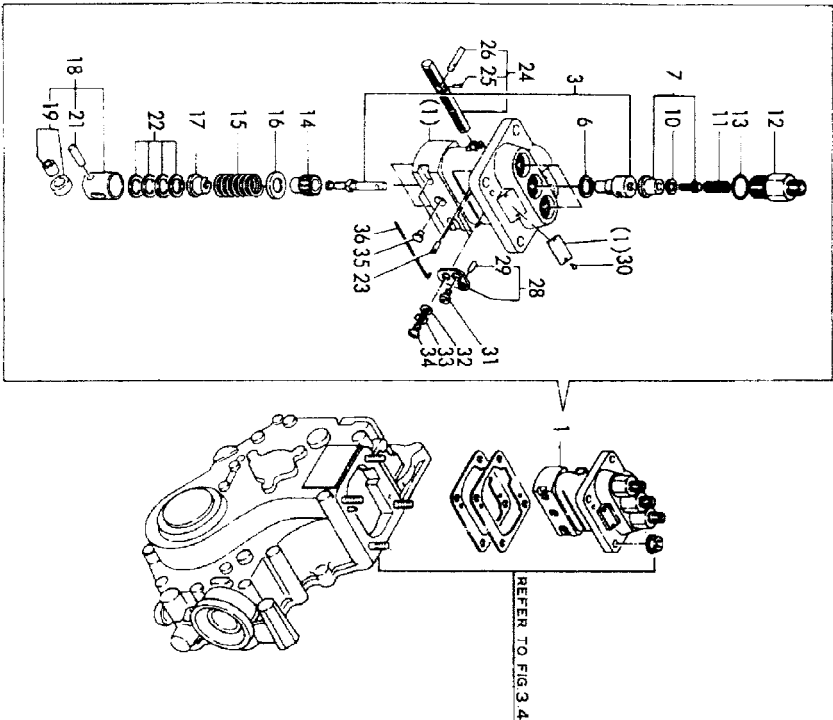
Fig.43 燃料噴射ポンプ FUEL INJECTION PUMP
