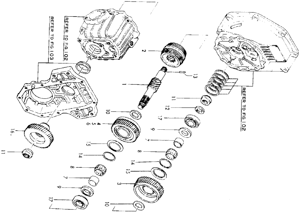
Fig. 106 出力シャフト OUTPUT SHAFT
