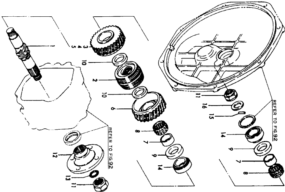
Fig. 94 OUTPUT SHAFT
