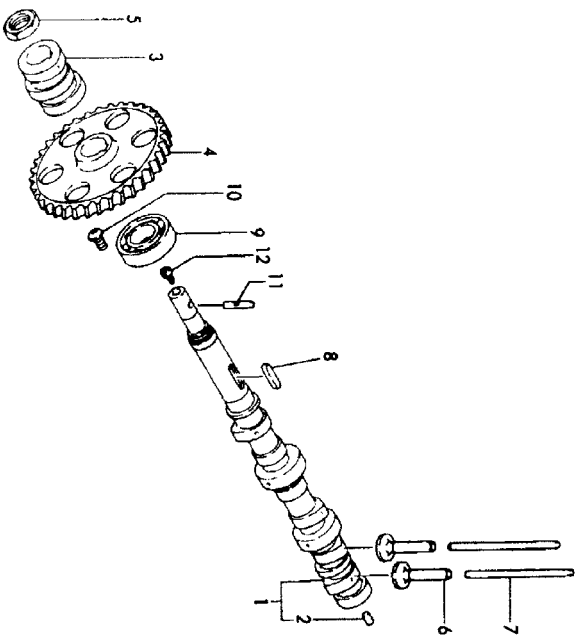
Fig.22 カムシャフト CAMSHAFT
