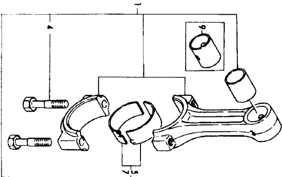
図.26 コネクティングロッド CONNECTING ROD
