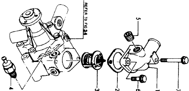
Fig.41 サーマスタット THERMOSTAT
