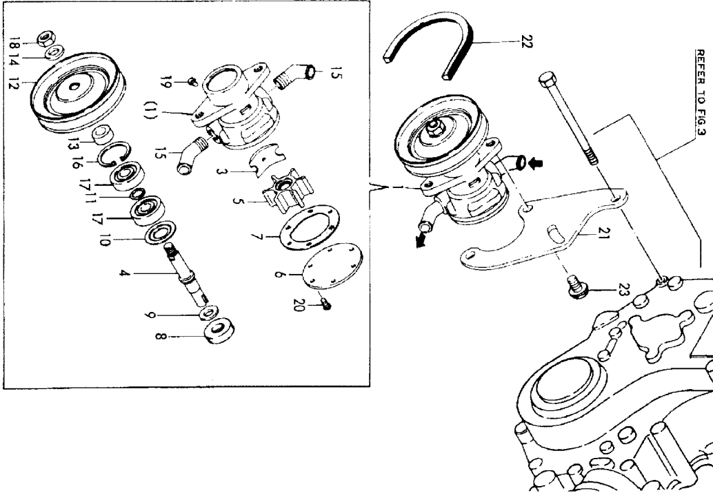
Fig.32 冷却水ポンプ(海水) COOLING SEA WATER PUMP
