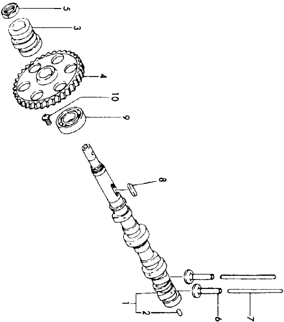
Fig.23 カムシャフト CAMSHAFT
