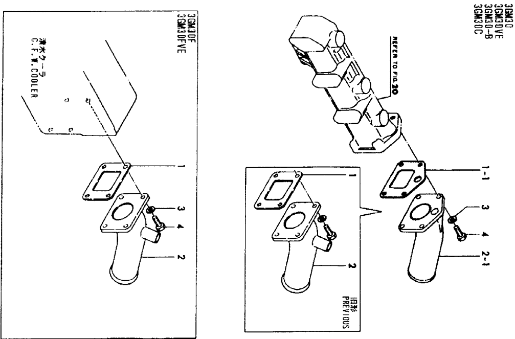
Fig. 21 ミキシングエルボ MIXING ELBOW
