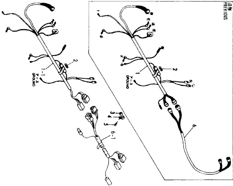
ワイヤハーネス 63 WIRE HARNESS
