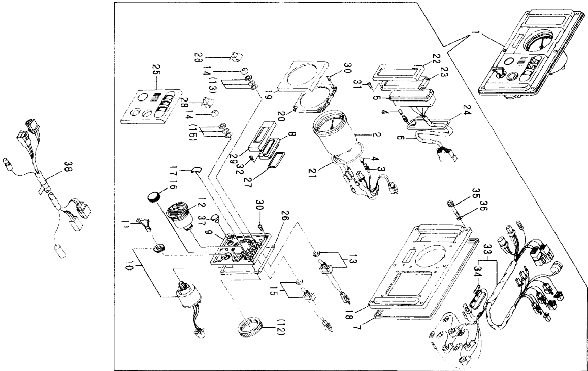
Fig. 85 計器盤 (Bタイプ, 新形, オプション) INSTRUMENT PANEL (B-TYPE, NEW, OPTIONAL)
