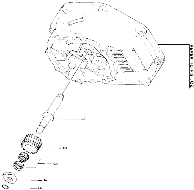
Fig. 105 サポートシャフト SUPPORT SHAFT
