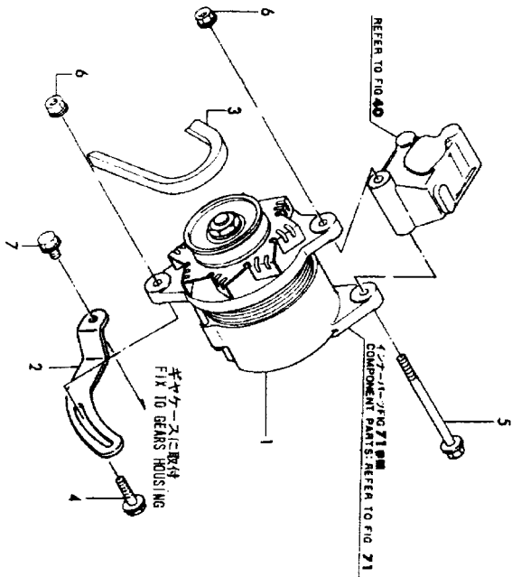
ジェネレータ Fig. 60 GENERATOR
