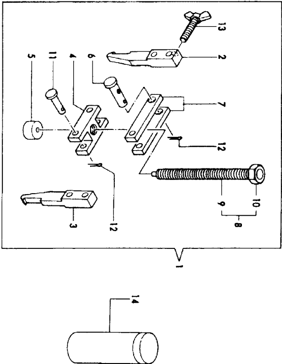
Fig. 101 工具(オプション) TOOL (OPTIONAL)
