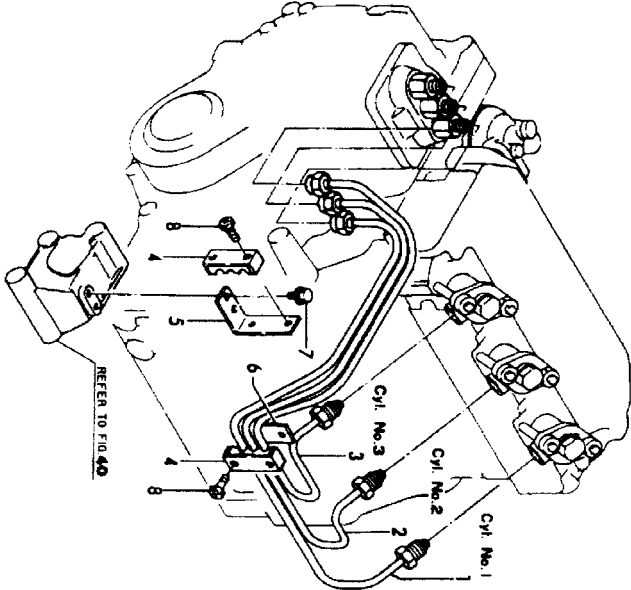
Fig.47 燃料噴射パイプ FUEL INJECTION PIPE
